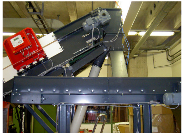
Verteilstation mit Metallabscheidung
